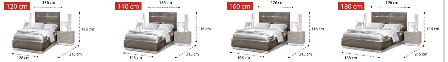
Letto LEGNO 120x200 LEGNO bed 120x200 Кровать LEGNO 120x200 Letto LEGNO 140x200 LEGNO bed 140x200 Кровать LEGNO 140x200 Letto LEGNO 160x200 LEGNO bed 160x200 Кровать LEGNO 160x200 Letto LEGNO 180x200 LEGNO bed 180x200 Кровать LEGNO 180x200
